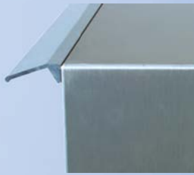
Bild 8: Regenschutzleiste, Alu-Profil
